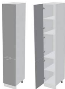
Корпус: ШП400-1 400x2140x553 (ШxВxГ) Фасад: ШП400-1 397x1317x16 (ШxВxГ) - 1 шт. 397x715x16 (ШxВxГ) - 1 шт.
