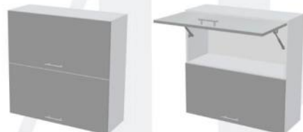
Корпус: ШВГ800 / ШВГС800 800x718x283 (ШxВxГ) Фасад: ШВГ800 797x356x16 (ШxВxГ) - 2 шт.
