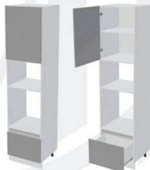
Корпус: ШП1Я600 600x2226x553 (ШxВxГ) Фасад: ШП1Я600 597x356x16 (ШxВxГ) - 1 шт. 597x715x16 (ШxВxГ) - 1 шт.
