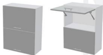
Корпус: ШВГ600 / ШВГС600 600x718x283 (ШxВxГ) Фасад: ШВГ600 597x356x16 (ШxВxГ) - 2 шт.
