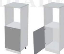
Корпус: ШПН600 600x1420x553 (ШxВxГ) Фасад: ШН1Д600 / ШНМ1Д600 / ШПН600 / ШВ1Д600 597x715x16 (ШxВxГ) - 1 шт.
