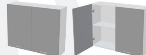
Корпус: ШВ1000 / ШВС1000 1000x718x283 (ШxBxГ) Фасад: ШВ1000 497x715x16 (ШxBxГ) - 2 шт.
