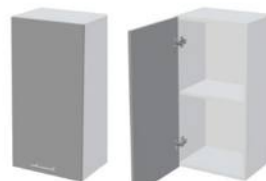
Корпус: ШВ400 / ШВС400 400x718x283 (ШxBxГ) Фасад: ШН400 / ШВ400 397x715x16 (ШxBxГ) - 1 шт.
