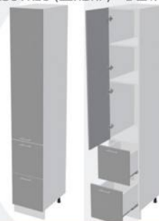
Корпус: ШП2Я400-1 400x2140x553 (ШxВxГ) Фасад: ШП2Я400-1 397x1317x16 (ШxВxГ) - 1 шт. 397x356x16 (ШxВxГ) - 2 шт.
