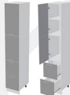
Корпус: ШП2Я400 400x2140x553 (ШxВxГ) Фасад: ШП2Я400 397x715x16 (ШxВxГ) - 1 шт. 397x597x16 (ШxВxГ) - 1 шт. 397x356x16 (ШxВxГ) - 2 шт.
