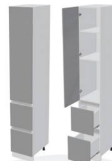
Корпус: ШП2Я400-1 400x2226x553 (ШxВxГ) Фасад: ШП2Я400-1 397x356x16 (ШxВxГ) - 2 шт. 397x1317x16 (ШxВxГ) - 1 шт.
